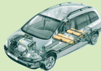
Platzierung der Erdgastanks
