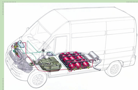
Platzierung Erdgastanks
